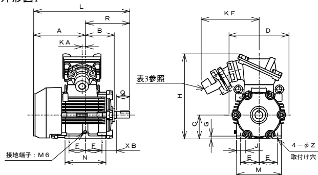
外形図1
