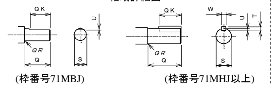
軸端詳細図
